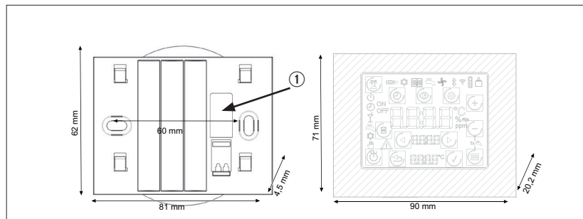
obr. 3.1 Nástěnný držák
